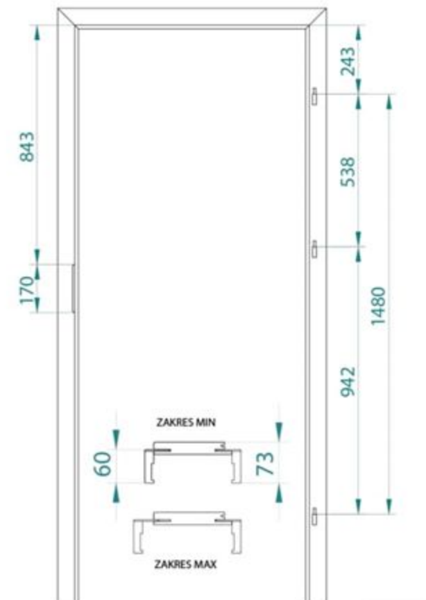
OŚCIEŻNICA REGULOWANA DO DRZWI PRZYLGOWYCH
