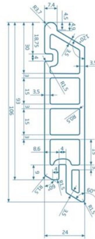
PROFIL ELEWACYJNY 106 X 24 MM
