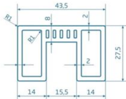
DASZEK NA SŁUPEK 60 X 60 MM
