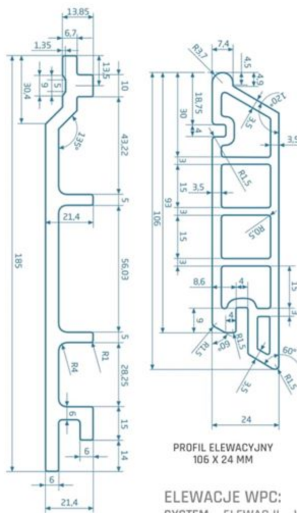
PROFIL ELEWACYJNY 185 X 20,4 MM
