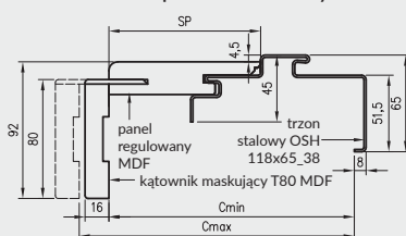
profil ościeżnicy
