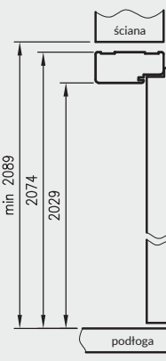
Przekrój pionowy drzwi przylgowych
