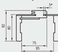
Przekrój ORB 075
