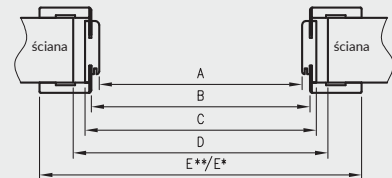
Przekrój poziomy OR/ORC
